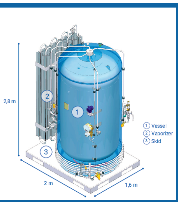
Skid Tank 3000 L 16 barg to 32 barg (PED compliant) Skid Tank 3000 L 16 barg đến 32 barg (Tuân thủ PED)
